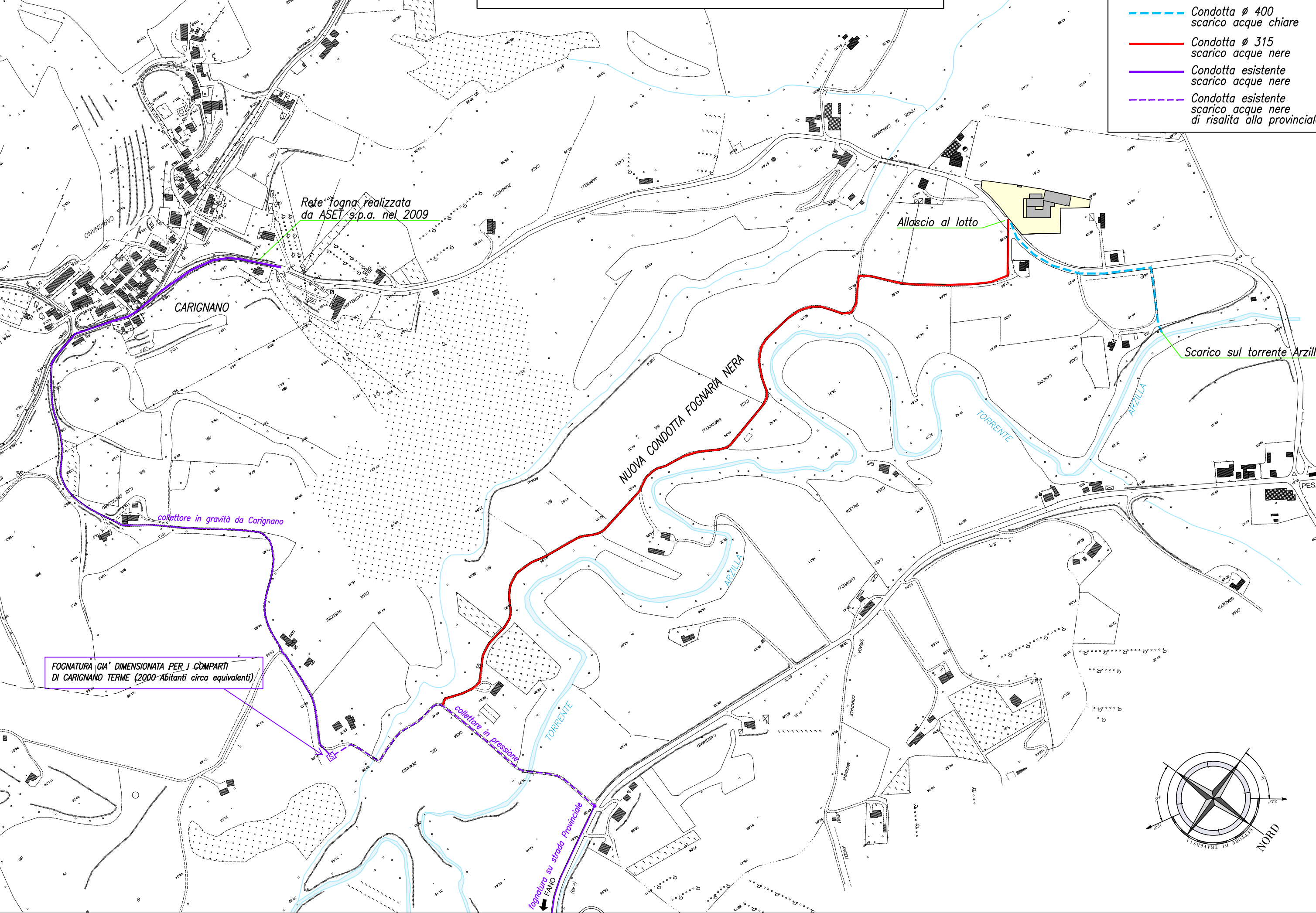
ESTRATTO CATASTALE CON INDICAZIONE DELLE PROPRIETÀ E DEI TRACCIATI DELLE FOGNATURE
