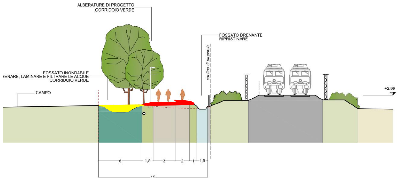
Figura 27 – In rosso: volumi sottratti alle esondazioni del fiume Metauro dal rilevato della ciclovia. In giallo: volumi di scavo a compensazione dei volumi sottratti (vasche di laminazione della ciclovia)
