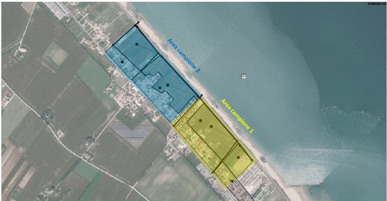
Figura 32 – Schema della rete nel modello SWMM nelle aree a campione selezionate
