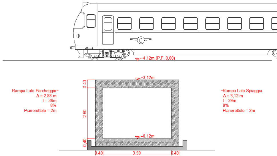
Figura 17: Sezione scatolare e rampe d'accesso del sottopassaggio ciclabile.
