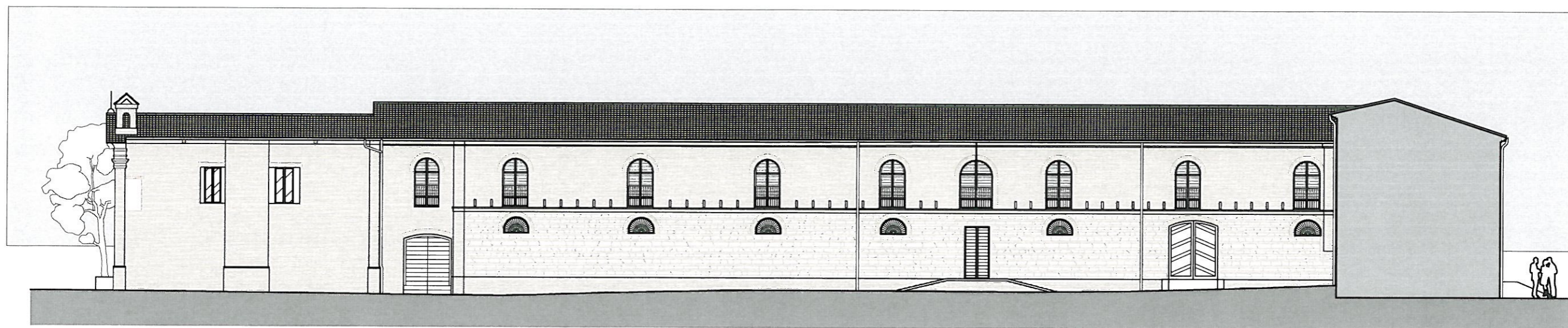
FIANCO DESTRO INTERNO SCALA 1:200
