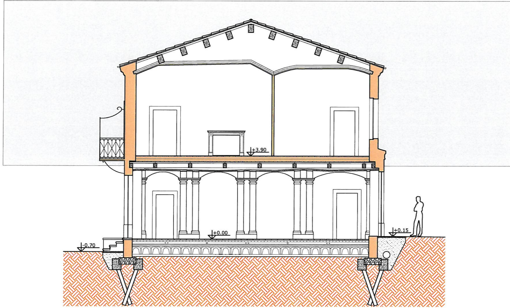
SEZIONE D-D' SCALA 1:100
