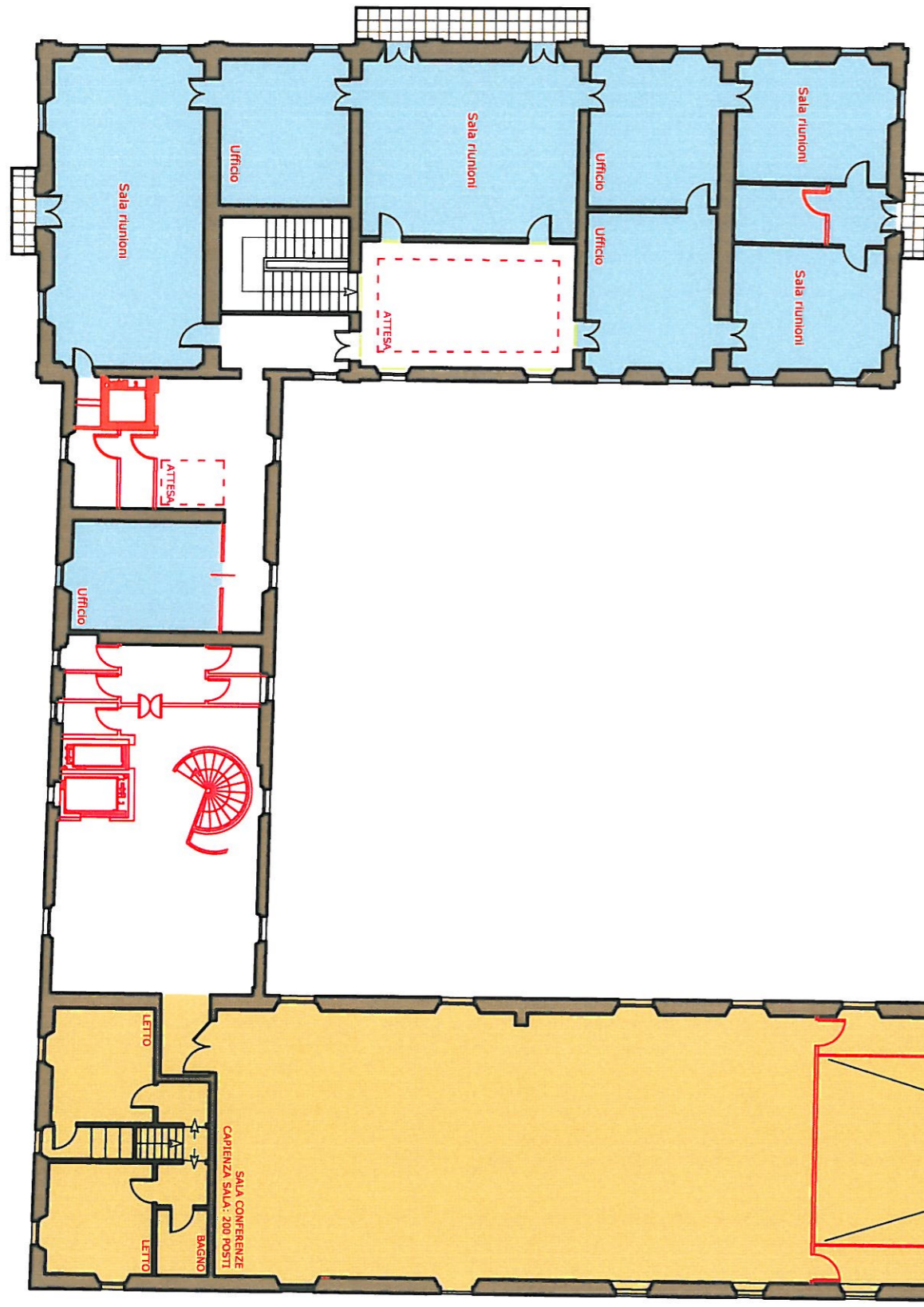
PIANO PRIMO SCALA 1:200
