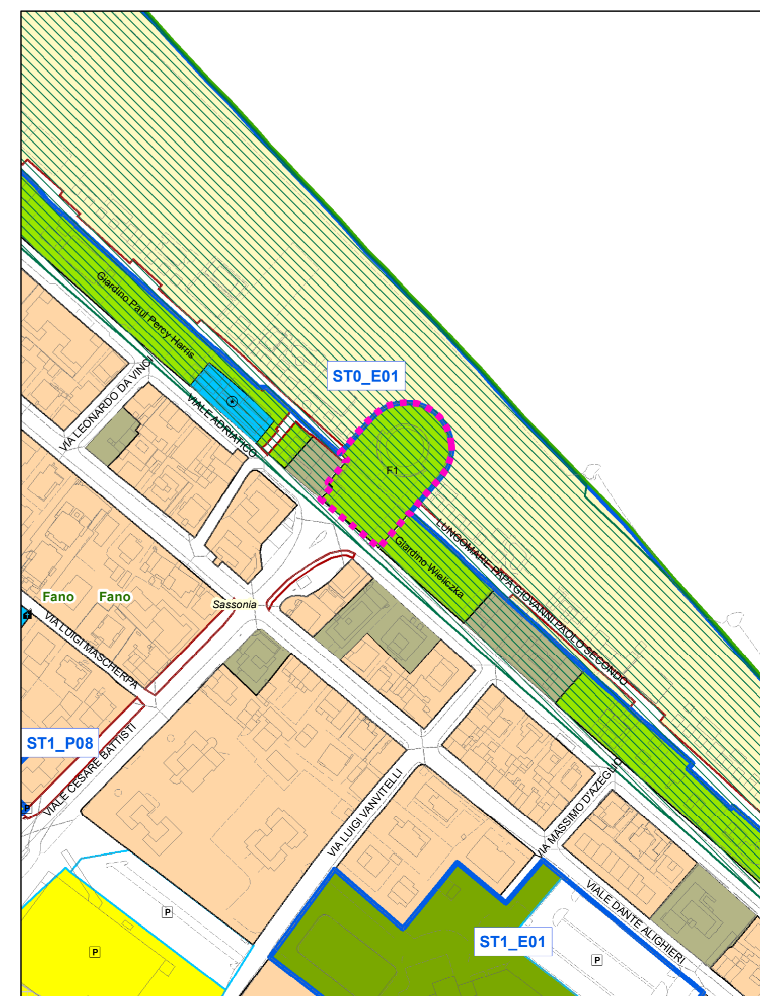
PRG VARIANTE - Progetto Urbanistico scala 1:2.000
