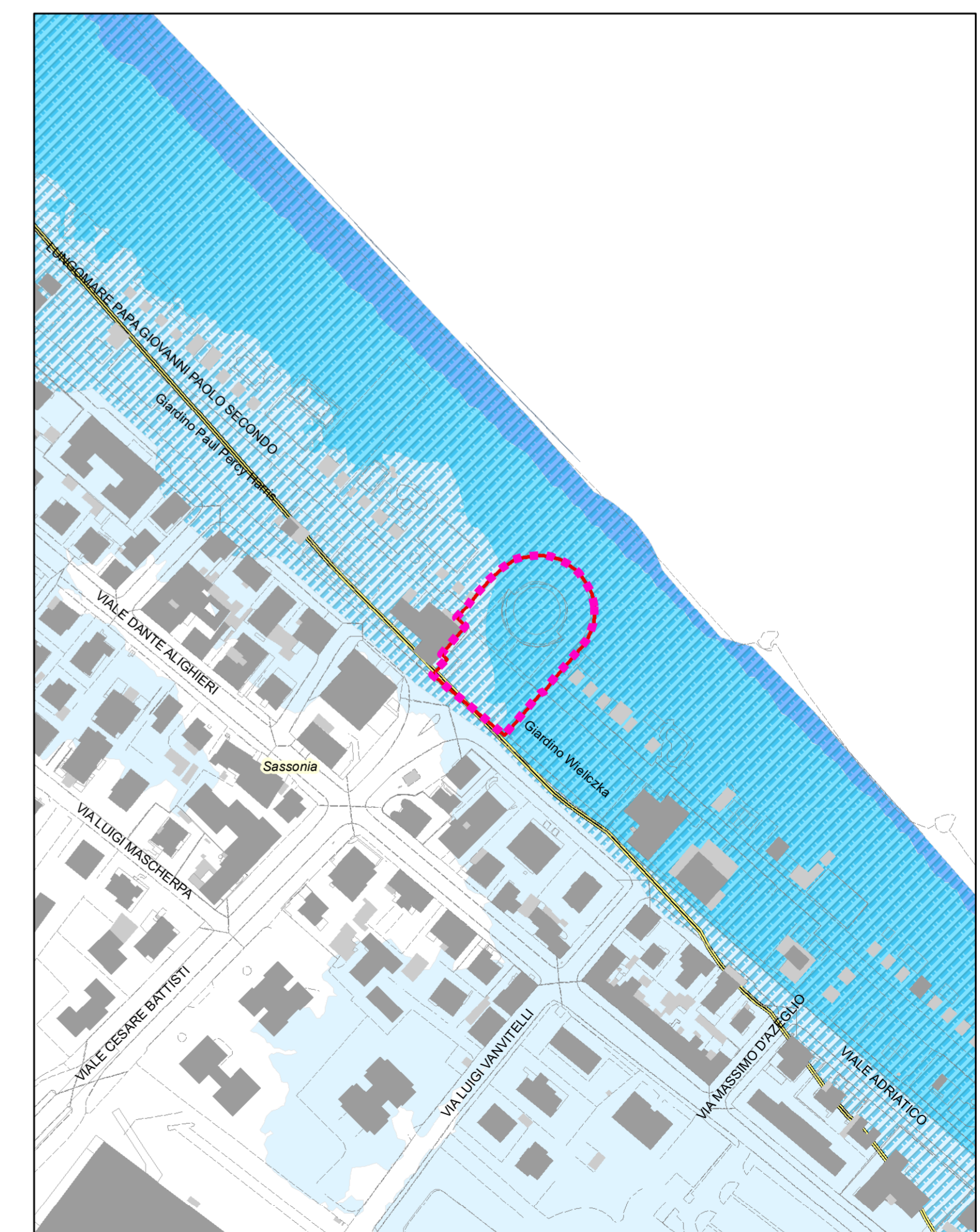
PRG VARIANTE - Ambiti di tutela scala 1:2.000
