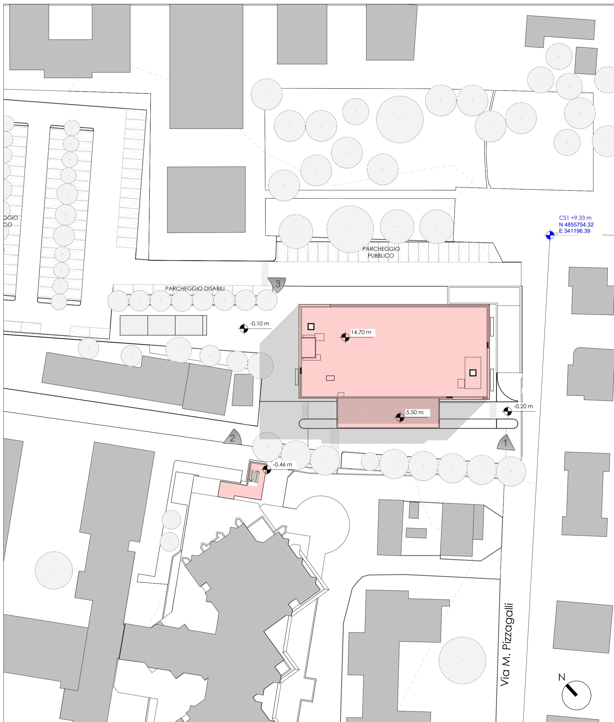
RILIEVO PLANIVOLUMETRICO scala [1:500]
