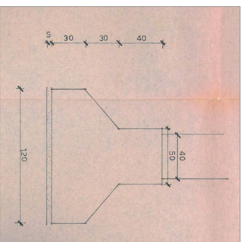
SEZIONE RICAVATA DAL PROGETTO ARCHITETTONICO
