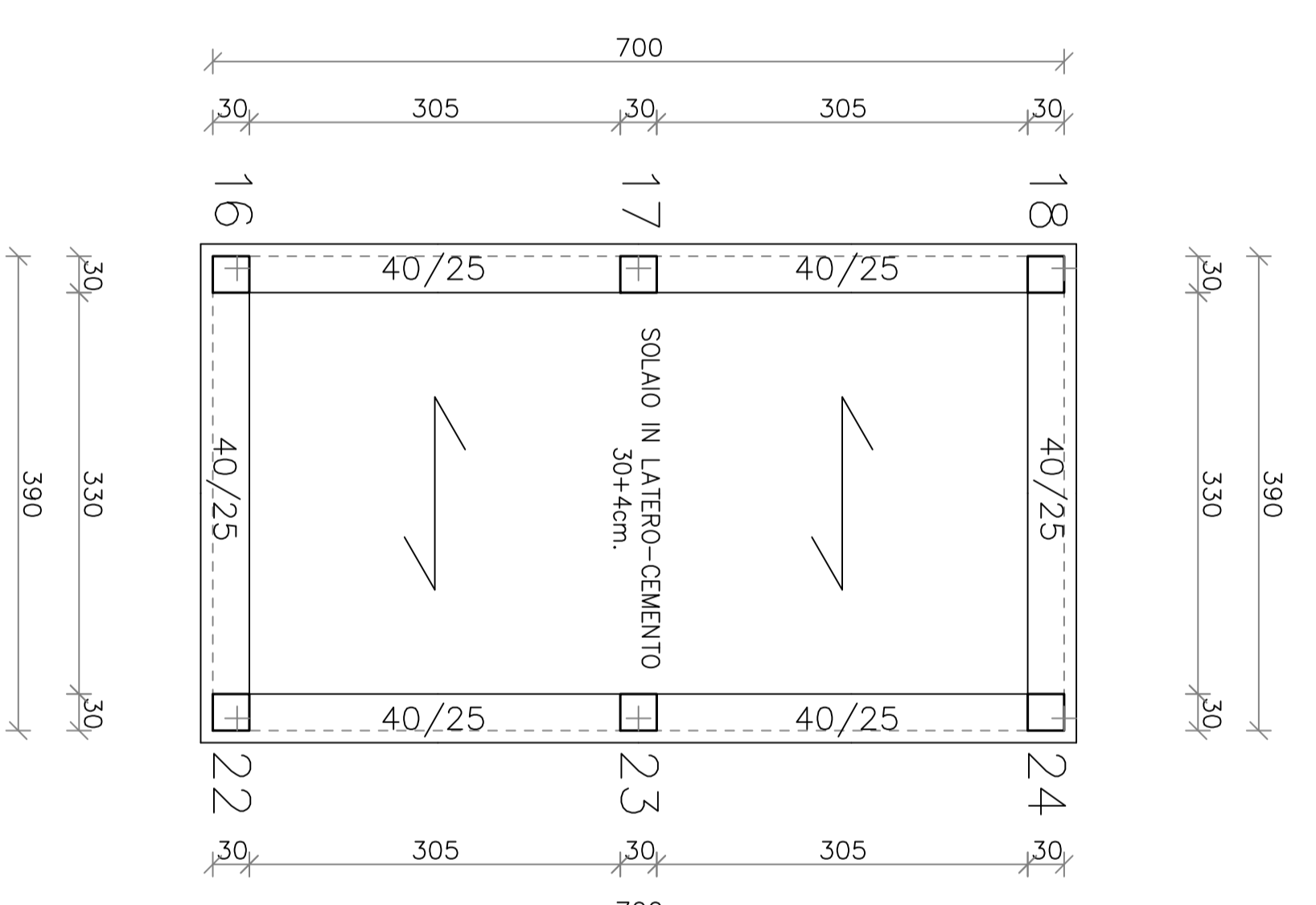
PIANTA DEL QUINTO SOLAIO – 1:50
