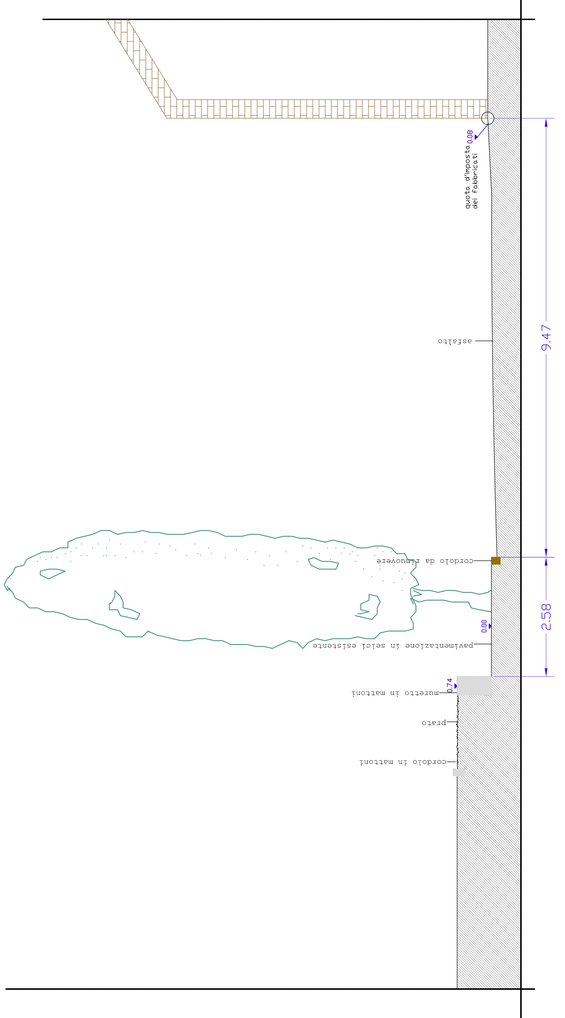
ATTUALE: VIA RIMEMBRANZE SEZIONE CC scala 1:50
