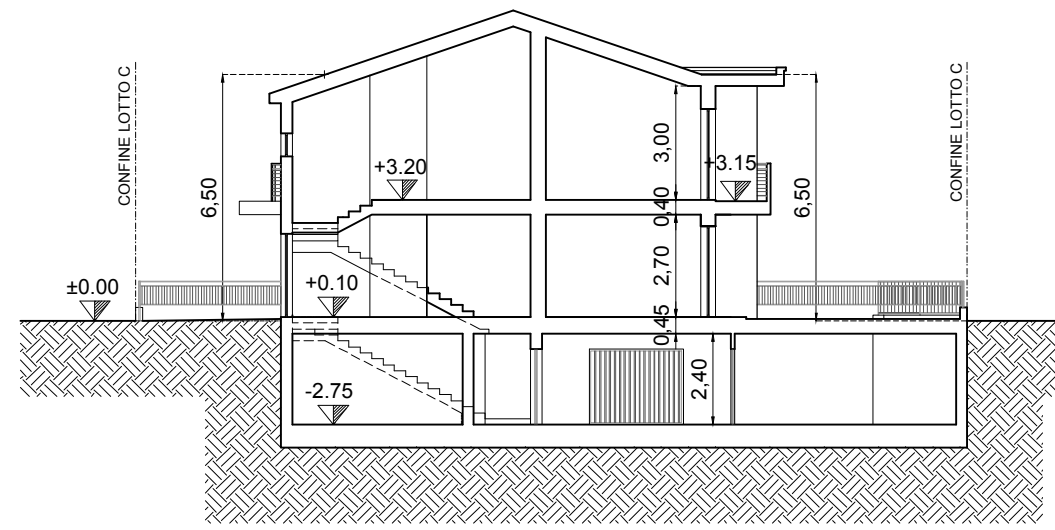
SEZIONE 1-1'
