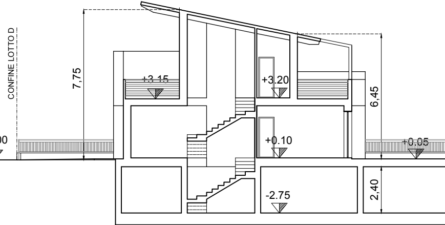
SEZIONE 2-2'
