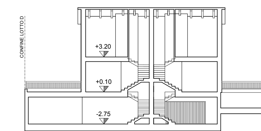
SEZIONE 1-1'
