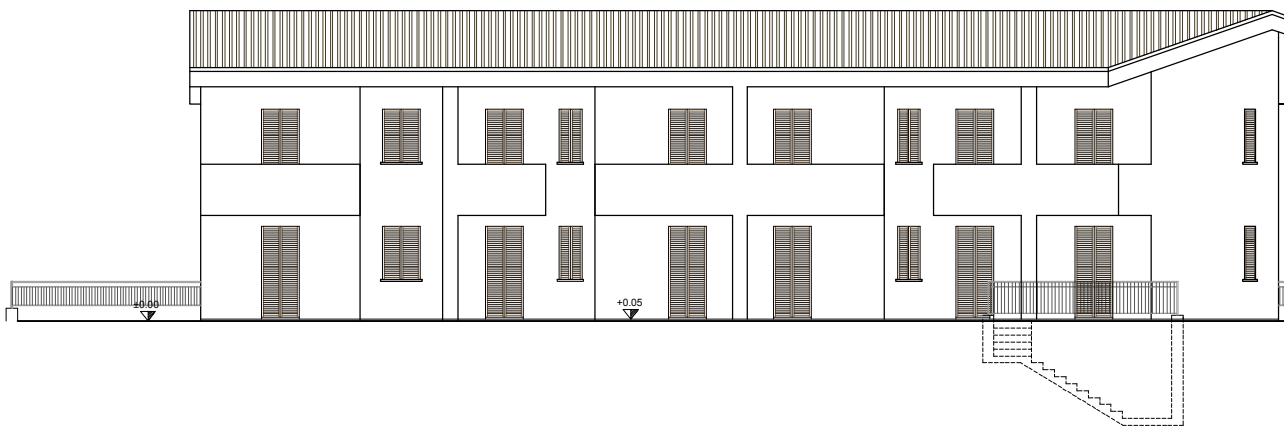
RETRO
