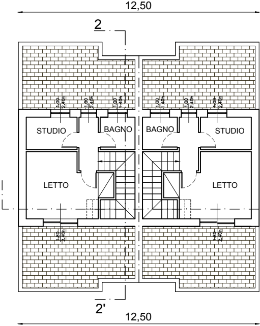
PIANO PRIMO
