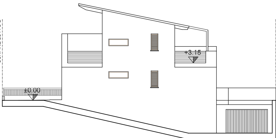
FIANCO DESTRO
