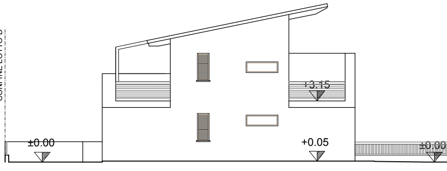
FIANCO SINISTRO
