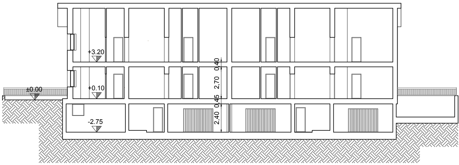
SEZIONE 2-2'
