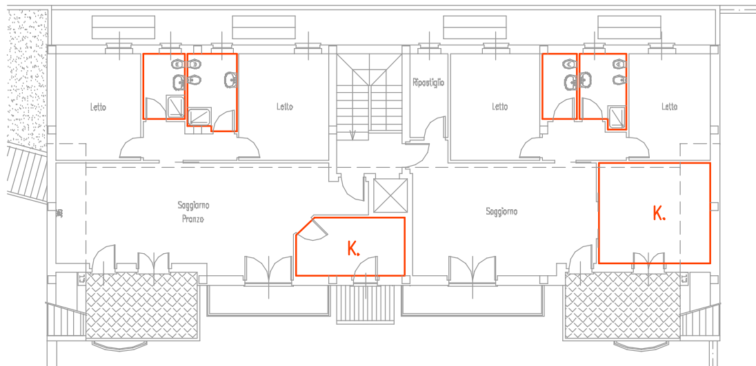
– PIANO SECONDO – scala 1:200
