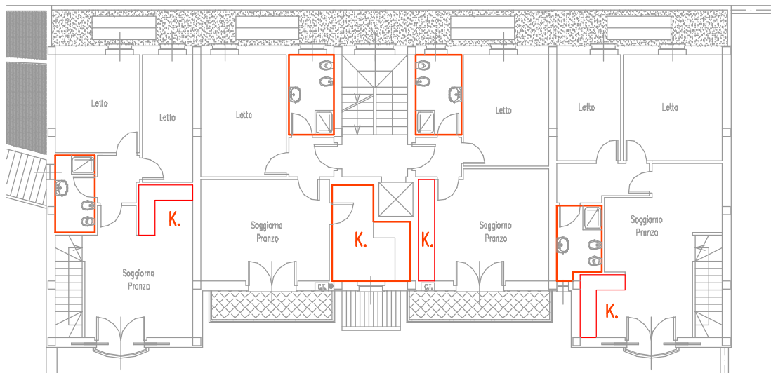
– PIANO PRIMO – scala 1:200
