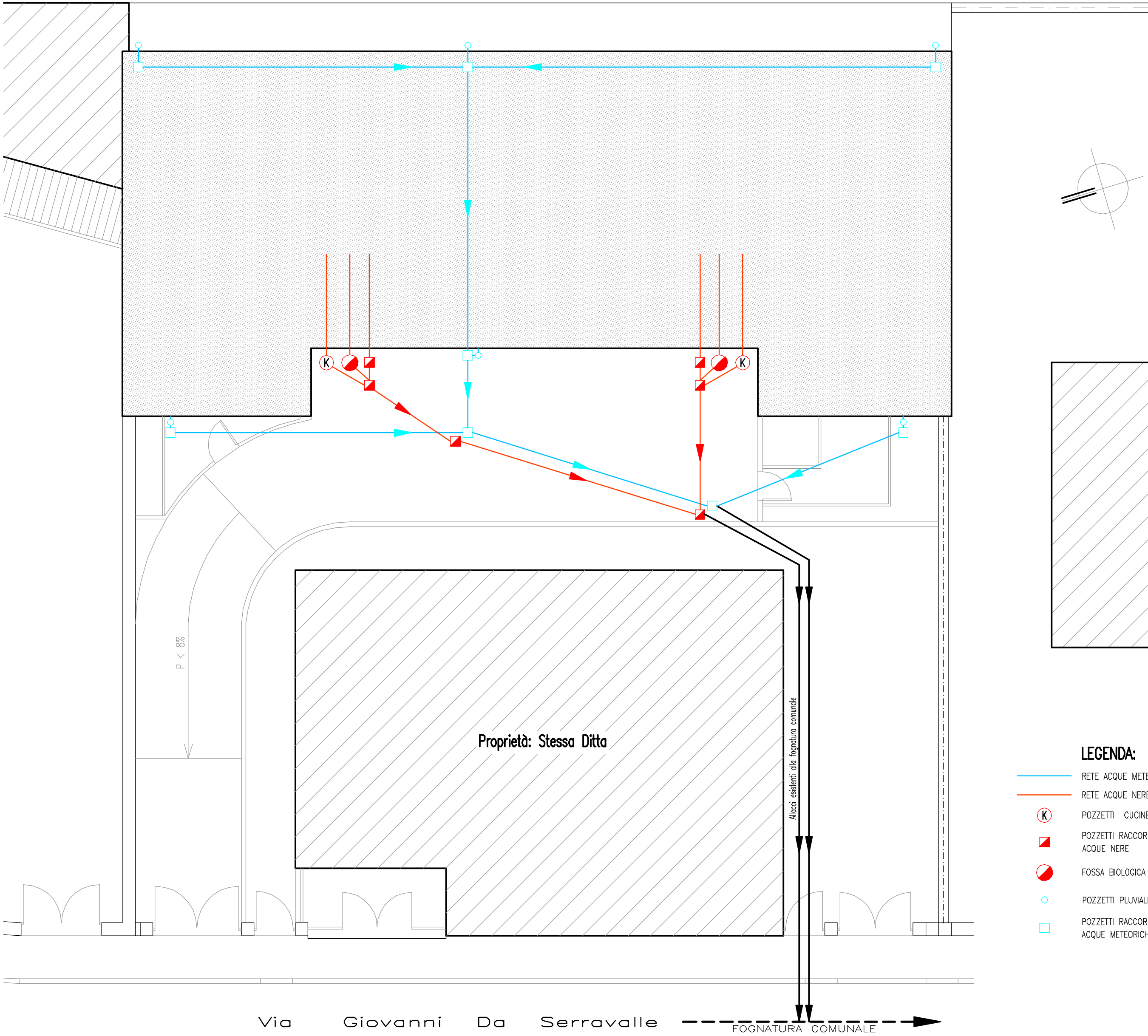
SCHEMA FOGNATURE scala 1:100
